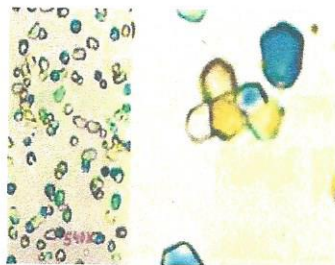
CALCIT-MIKRO-KRISTALL RasterElektronen-Mikroskop-Foto als Beweis für das Abrasions-Potenzial
